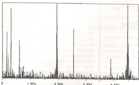
Fig. 4 : « Spectre des fréquences pour une autre partie de l'impulsion J confirme l'apparition de différences de fréquences identiques et égales à une des fréquences fondamentales. ».
