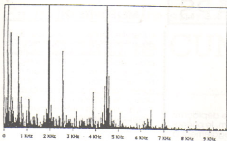
Fig. 3 : Le spectre des fréquences dans l'impulsion J présente des raies, comme un système qui ne peut vibrer qu'à certaines fréquences propres. »
